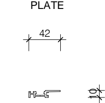
PAS509/T DOOR SEAL RAIL
