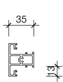
PAS 505 45 45MM MID RAIL
