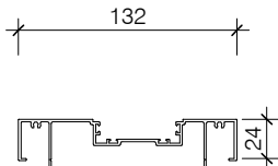
PAS535 132 DOOR STOP FRAME
