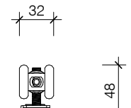
200KG ROLLER PACK OPTIONAL 120/160KG SOFT-CLOSE
