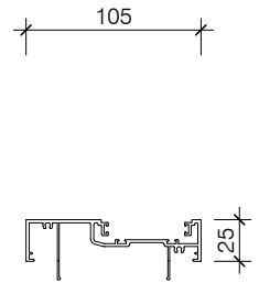
PAS533 105 DOOR STOP FRAME
