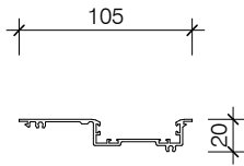
PAS 533/C DOOR STOP FRAME
