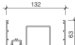
PAS555 BI-FOLD DOOR HEAD FRAME
