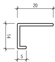
9MM EDGELINE 467371
