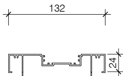
PAS535 132 DOOR STOP FRAME
