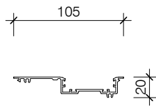
PAS 533/C DOOR STOP FRAME
