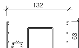
PAS555 BI-FOLD DOOR HEAD FRAME
