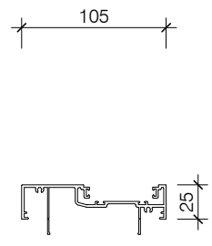
PAS533 105 DOOR STOP FRAME
