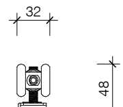
200KG ROLLER PACK OPTIONAL 120/160KG SOFT-CLOSE
