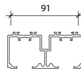
PAS522/D DS SLIDING DOOR TRACK
