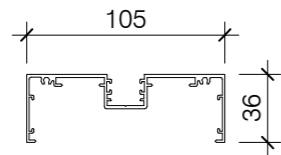
PAS015 POCKET MULLION / DOOR FRAME
