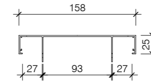
PAS310/DD HEAD TRACK DOUBLE DOUBLE
