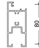
PAS503/80 DS DOOR RAIL 80MM
