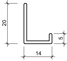
467371 9MM EDGE LINE
