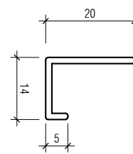
9MM EDGELINE 467371
