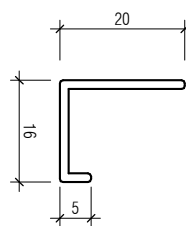
12MM EDGE LINE 467372
