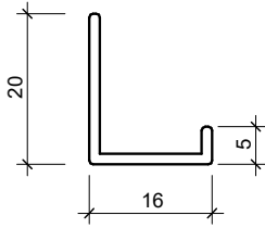
467372 12MM EDGE LINE
