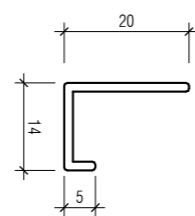
9MM EDGELINE 467371
